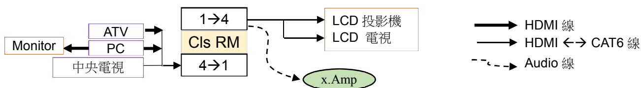
課室 HDMI 設備連接簡圖
